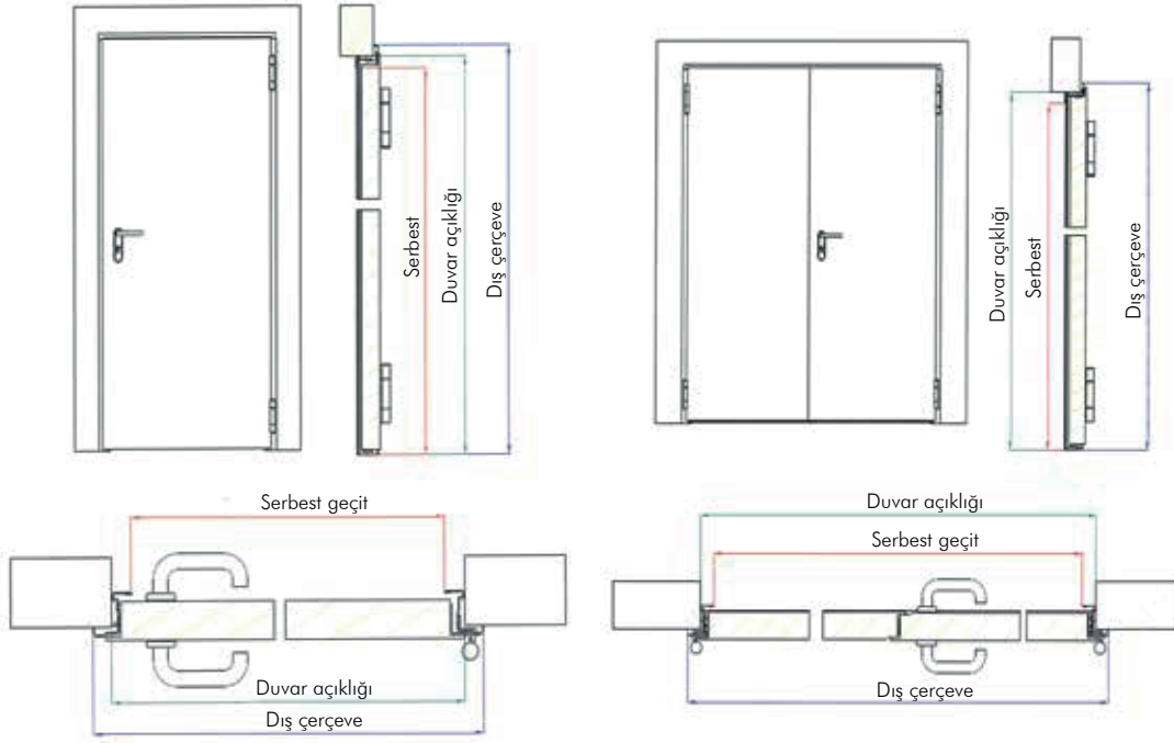
ÇERÇEVE + ÖN ÇERÇEVE+ KAPI GİRİŞİ
